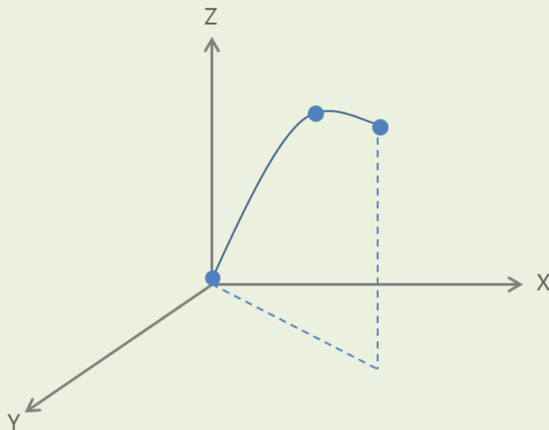
&lt; 3축 스플라인 보간 이송 &gt;
