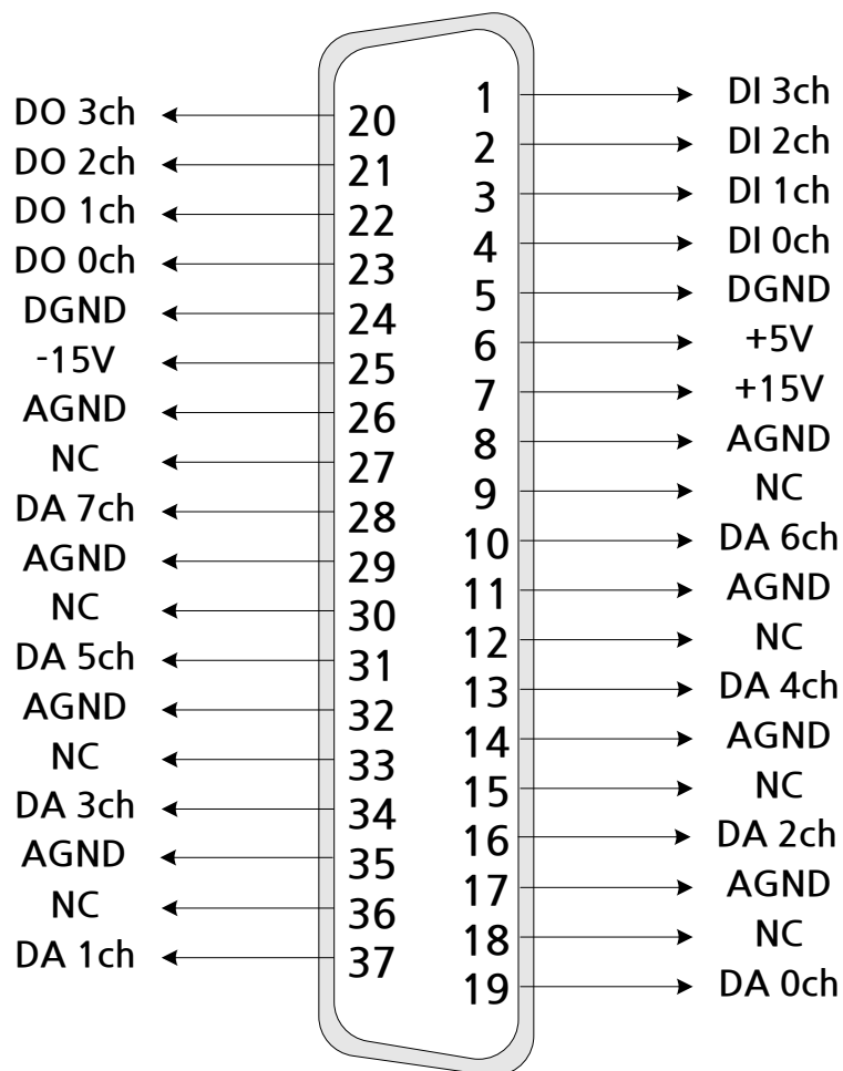
[그림 1-3] COMI-CP302 커넥터 핀 배열
