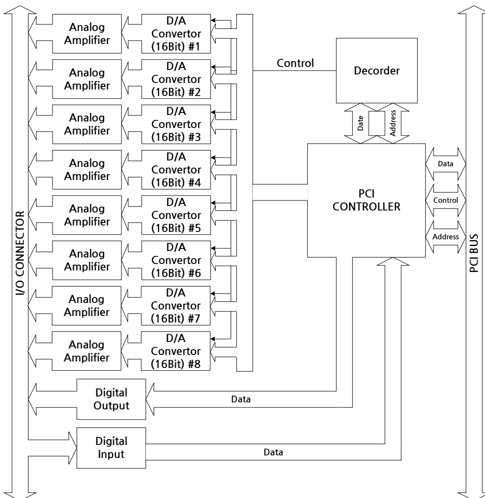
[그림 1-2] COMI-CP302 Hardware 개념도
